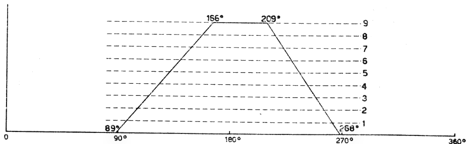
spostamento attuatori
