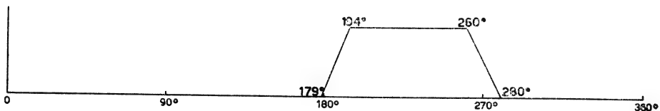
ingranamento dentierine
